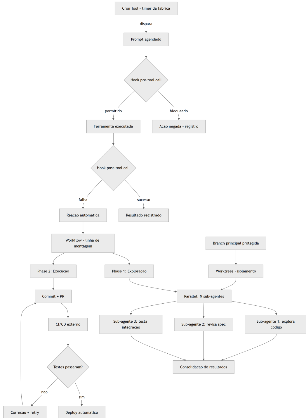
Figura 18: A fábrica de automação: cron, hooks, workflows e sub-agentes orquestrando a produção
