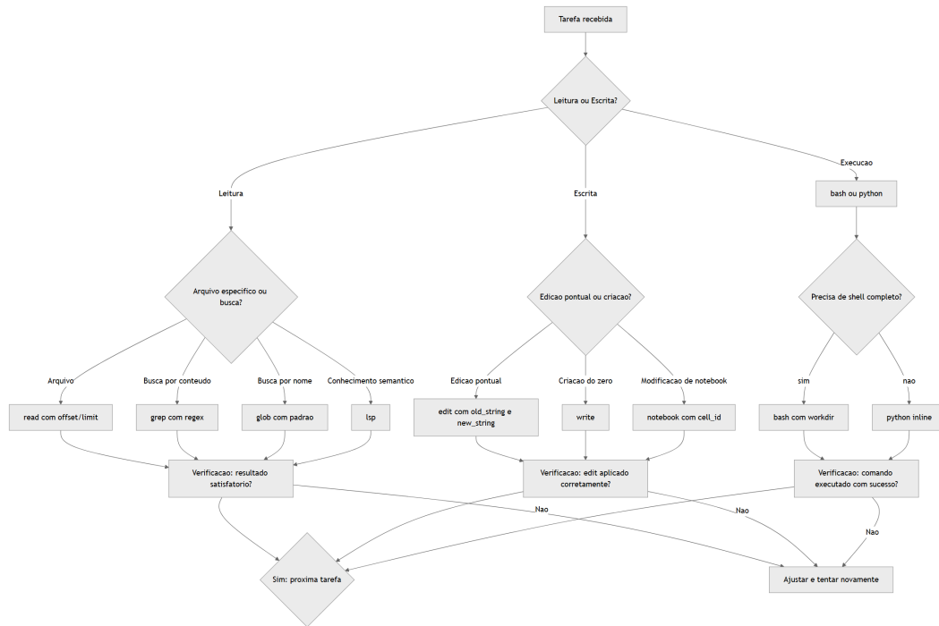
Figura 7: Fluxo de decisão do Oh My Pi para seleção de ferramenta
