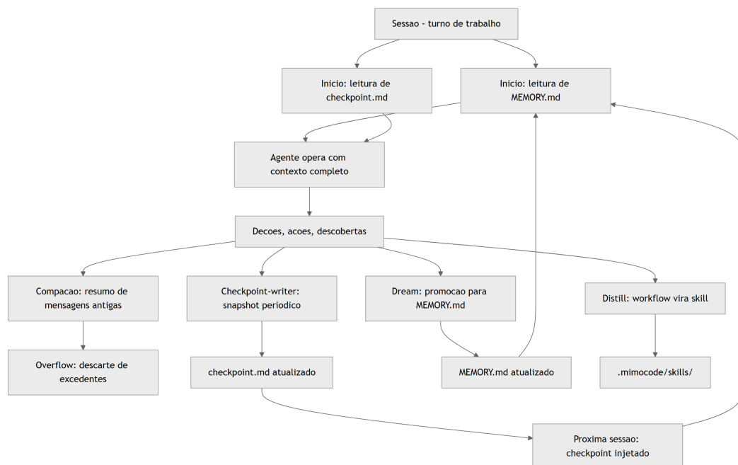
Figura 12: O sistema de memória do OMP como escritório com arquivos e turnos
