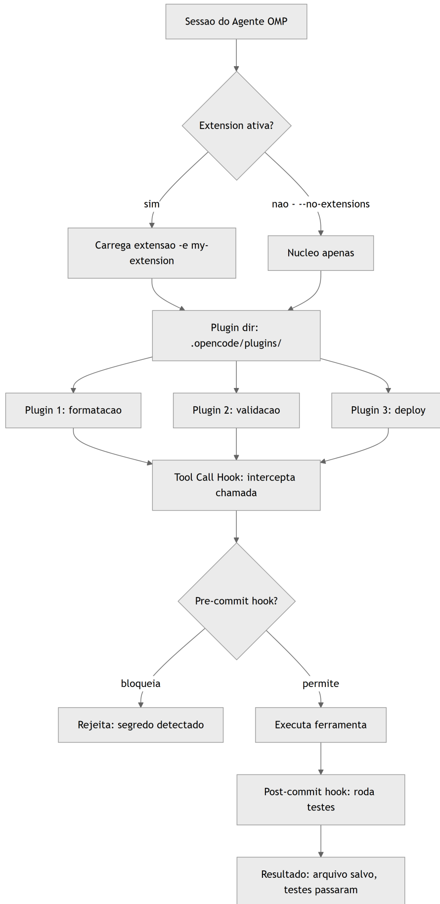
Figura 14: A oficina extensível: plugins, hooks e extensions no ciclo de vida do agente
