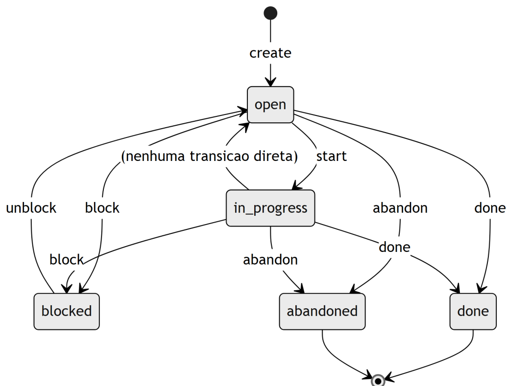
Figura 11: Máquina de estados do ciclo de vida de uma tarefa
