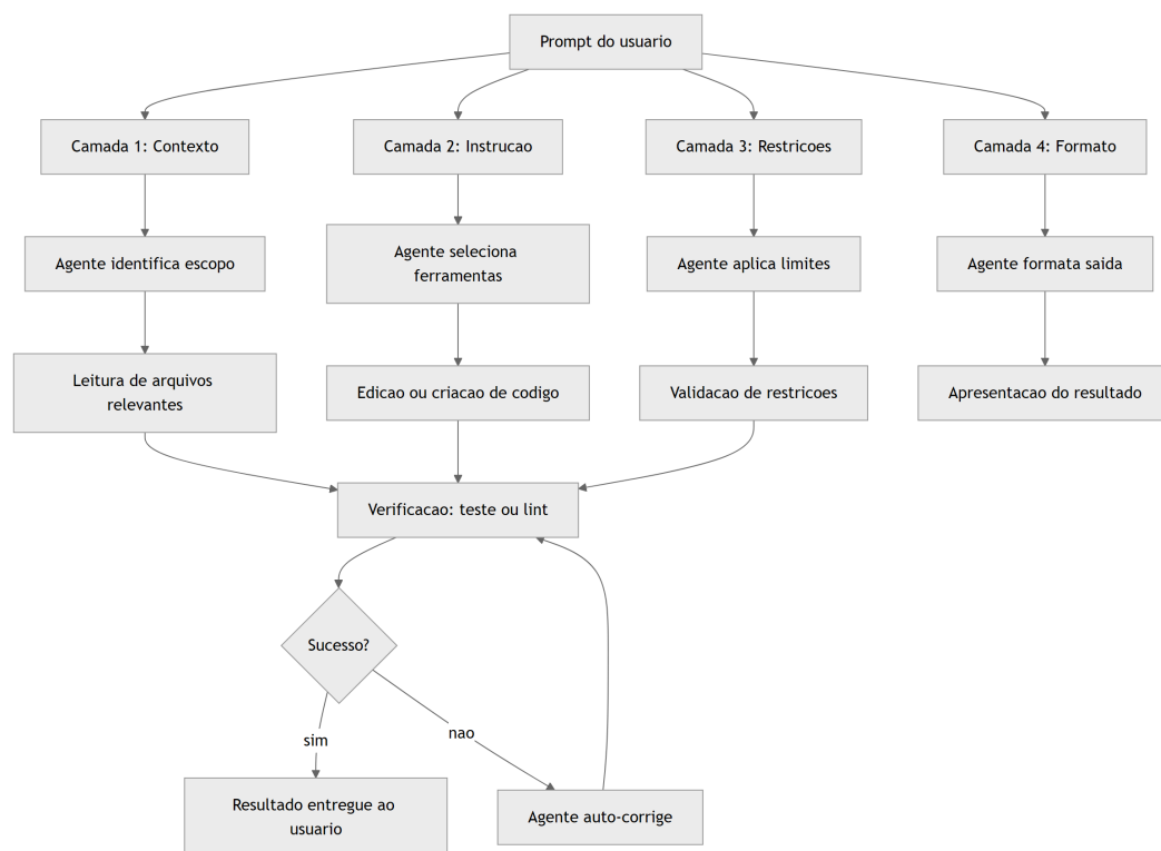
Figura 5: Fluxo de execução de um prompt no Oh My Pi — das quatro camadas à ação concreta
