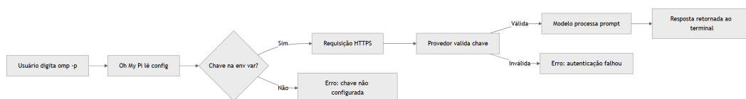
Figura 3: Fluxo de autenticação entre Oh My Pi e provedor de modelo
