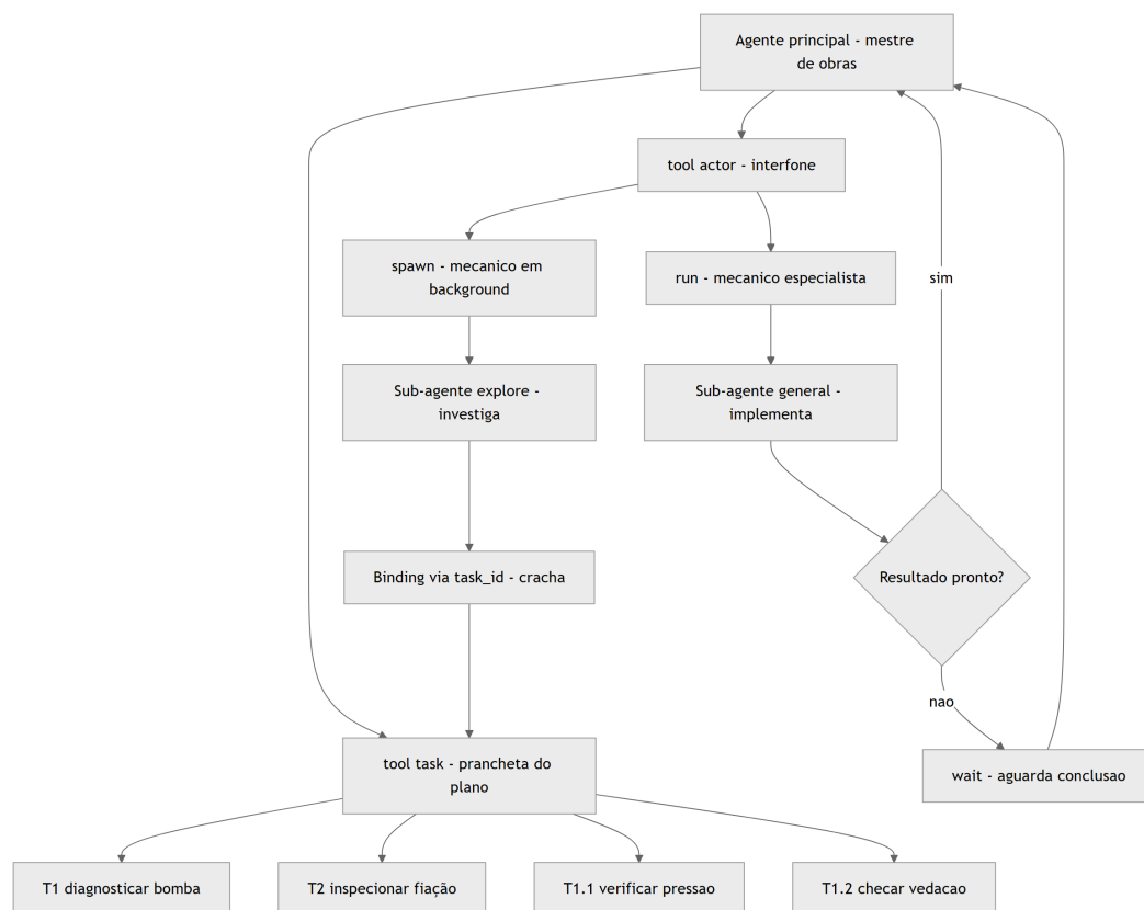
Figura 9: A oficina de orquestracao: mestre de obras despacha mecanicos por tarefa
